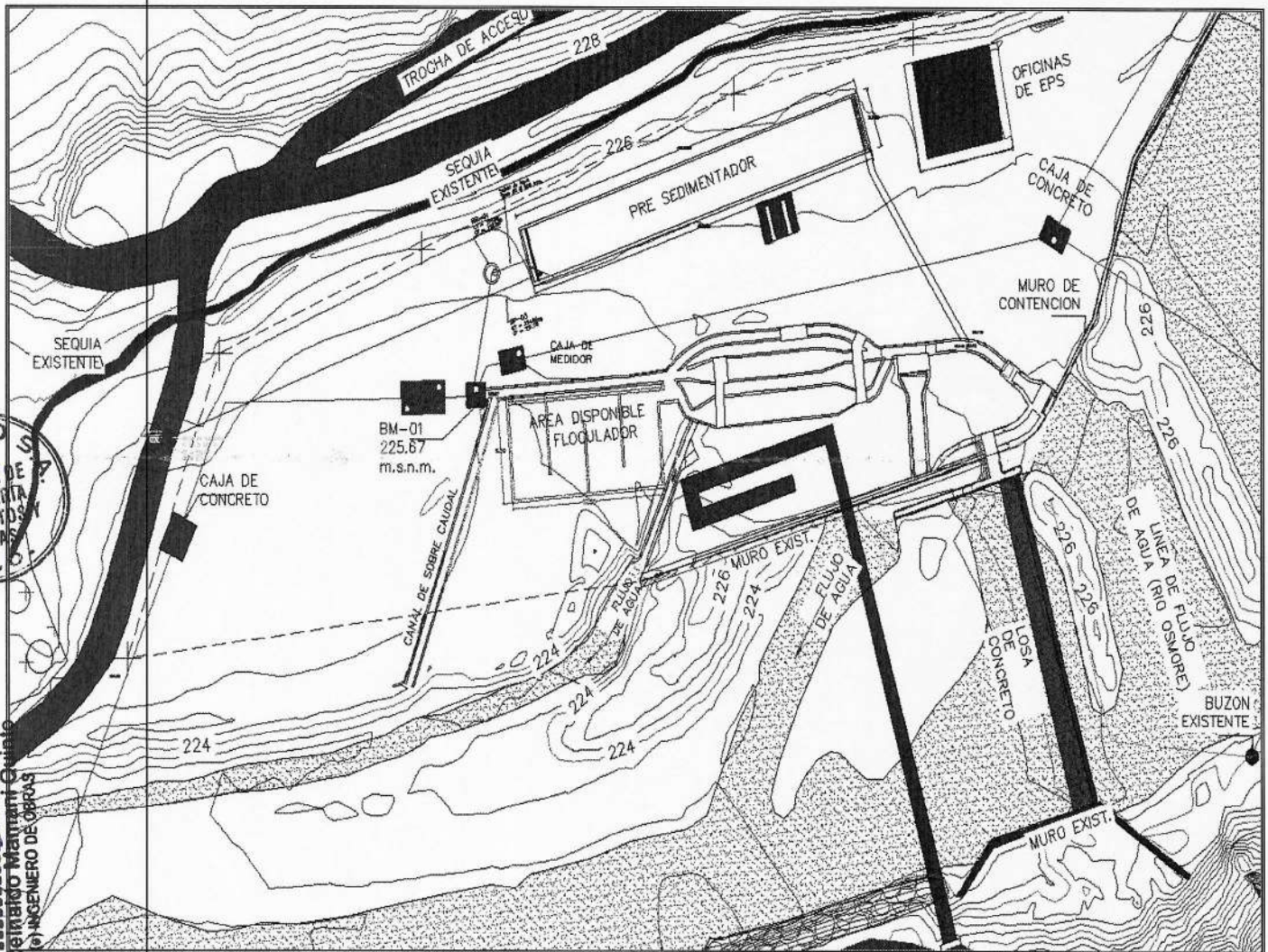
BOCATOMA DE CAPTACION PASTO GRANDE
