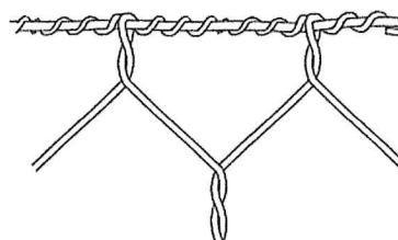
Detalle de la Unión Mecánica de la malla con el alambre de borde (S/E)
