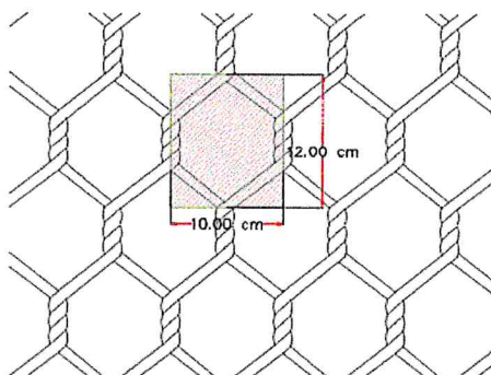
Detalle de las dimensiones de la cocada (S/E)
