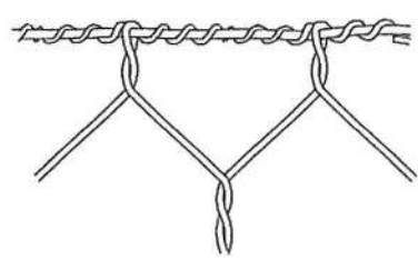
Detalle de la Unión Mecánica de la malla con el alambre de borde (S/E)
