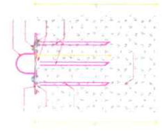
DETALLE 1 DE ANCLAJE ESC. 1:25
