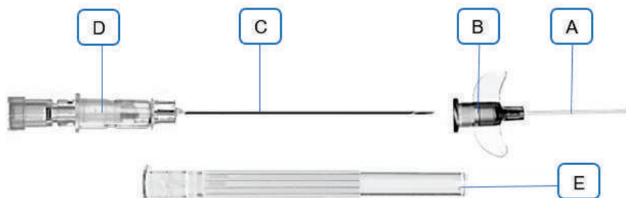
A: Catéter; B: Cono del catéter con alas; C: Aguja introductora; D: Dispositivo de bioseguridad con sistema de activación activo (mecánico); E: Protector Figura 2: Catéter endovenoso periférico con dispositivo de bioseguridad con sistema de activación activo (mecánico) y alas de fijación. (No incluye diseño)
