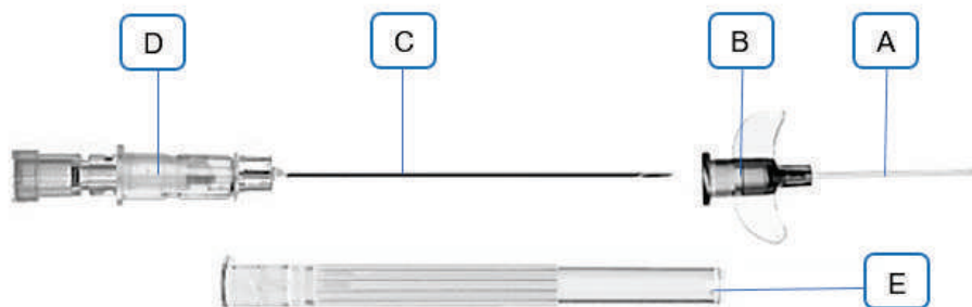
A: Catéter; B: Cono del catéter con alas; C: Aguja introducciona; D: Dispositivo de bioseguridad con sistema de activación activo (mecánico); E: Protector activo (mecánico) y alas de fijación. (No incluye diseño) Figura 2: Catéter endovenoso periférico con dispositivo de bioseguridad con sistema de activación activo (mecánico) y alas de fijación. (No incluye diseño)
