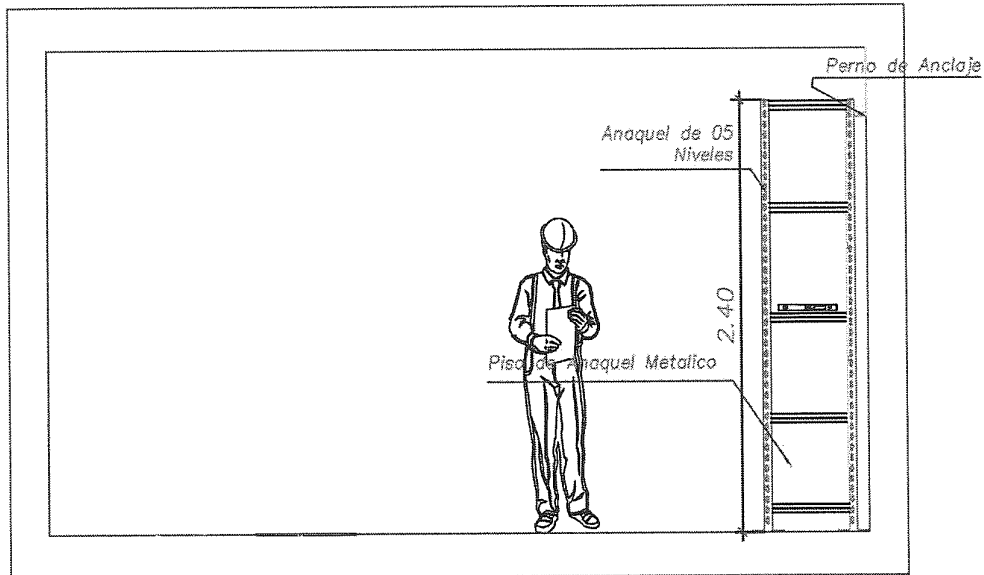
CORTE B-B
