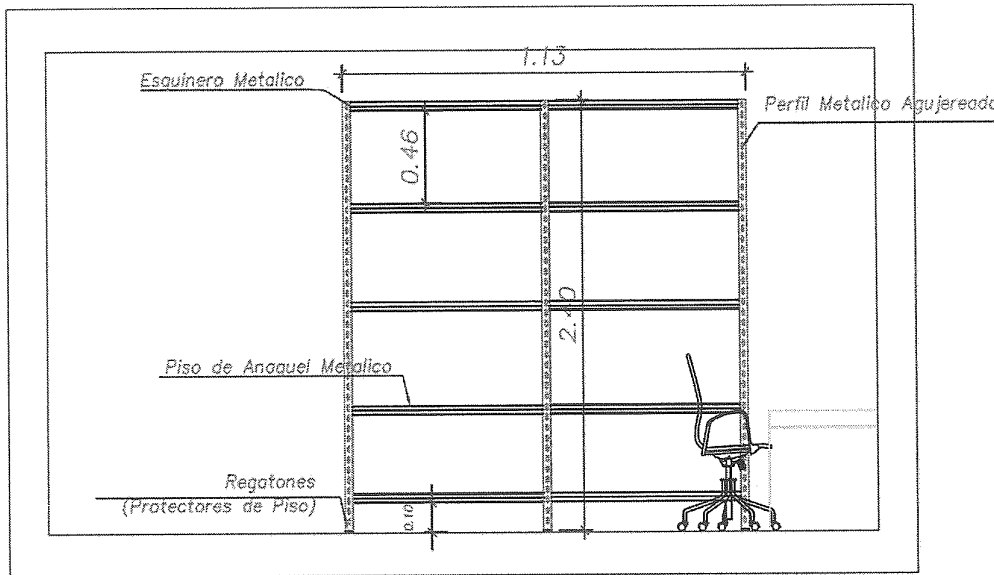
CORTE A-A
