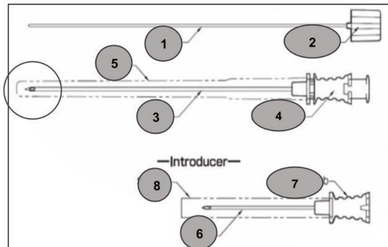
Fig. 1: Aguja de punción lumbar (no incluye diseño)
