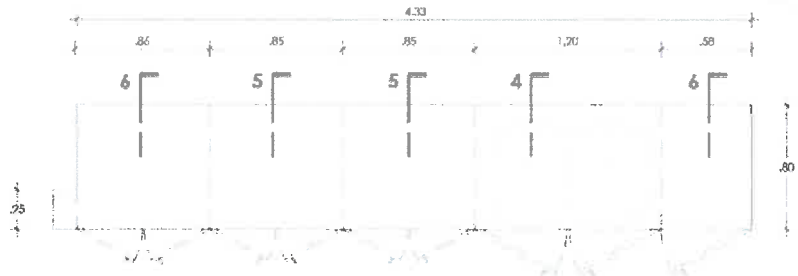
MB_LH 02 ESC. 1/20
