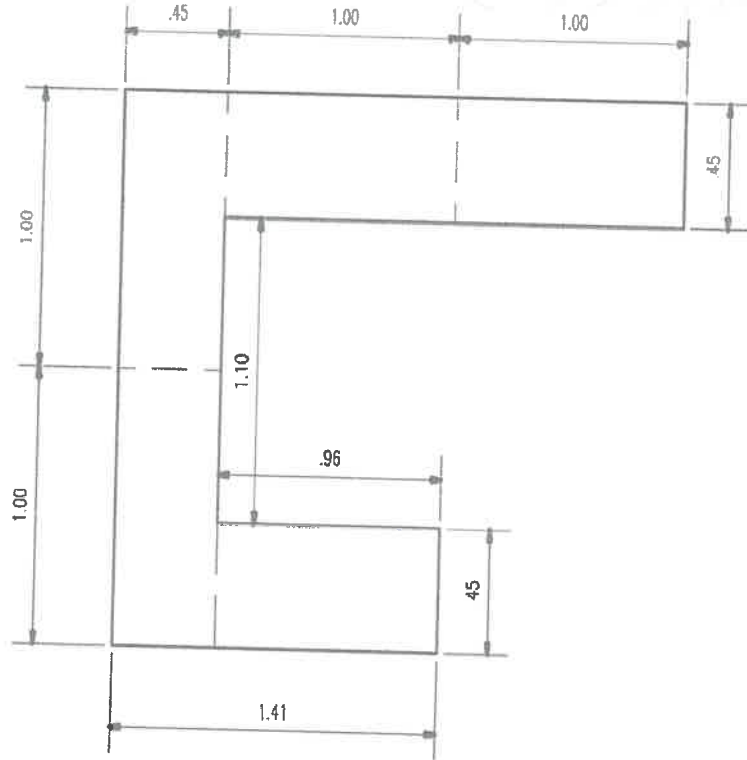
Plano en planta
