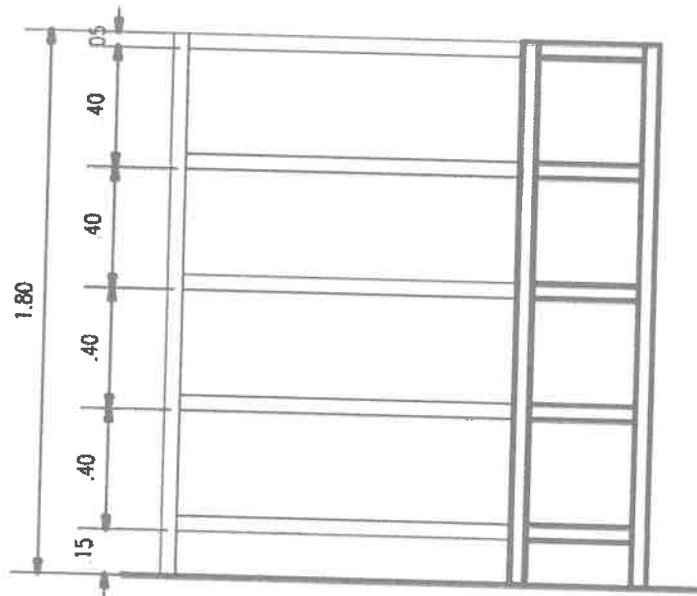
CORTE A-A ESC. 1/20
