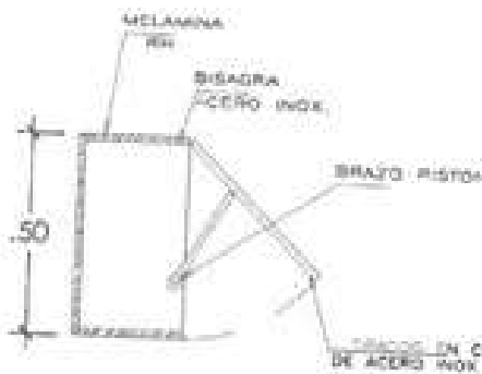
IMAGEN REFERENCIA DE BISAGRA CON BRAZO PISTON
