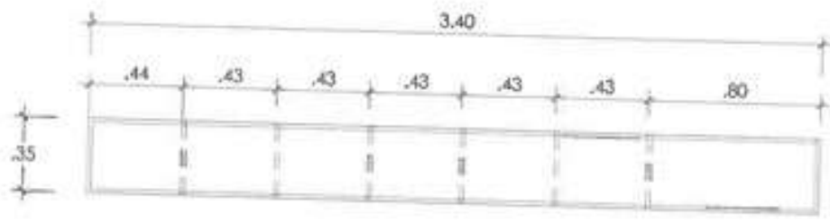
ESTANTE - VISTA EN PLANTA ESC. 1/20
