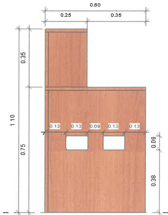
CORTE 1-1
