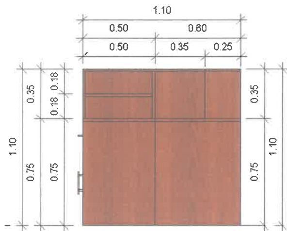
VISTA LATERAL
