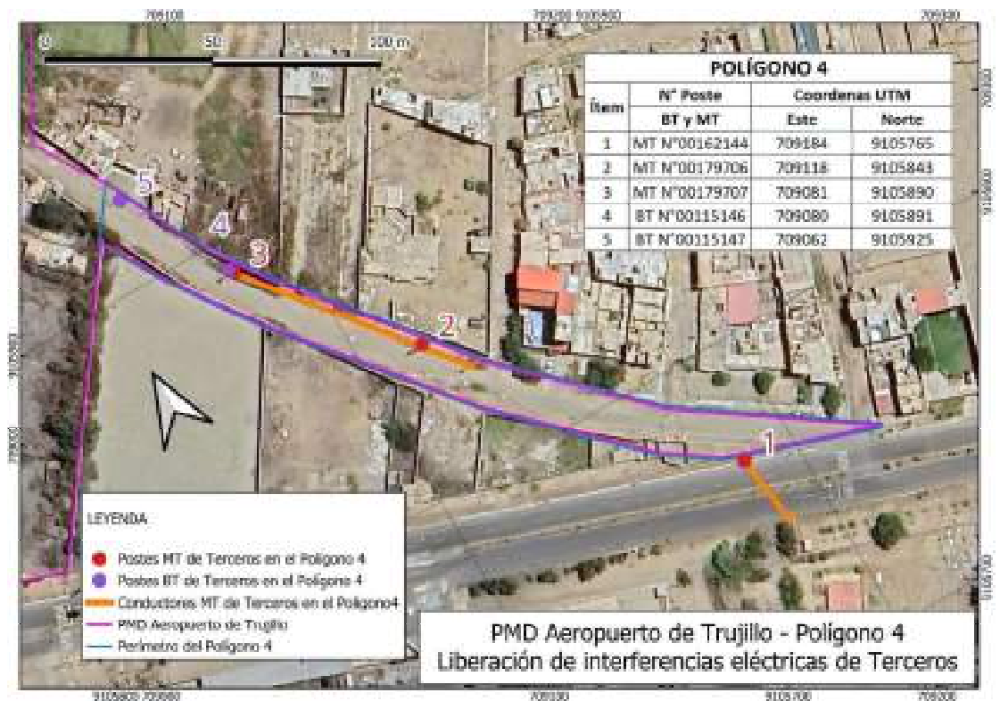
Figura 02: Ubicación de los postes de concreto de MT y BT más conductores MT de titularidad de Terceros para desmontaje o liberación de interferencia eléctrica.
