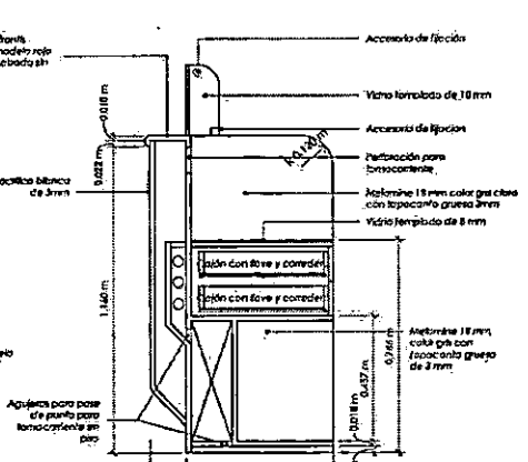
CORTE A-A ESC: 1/15
