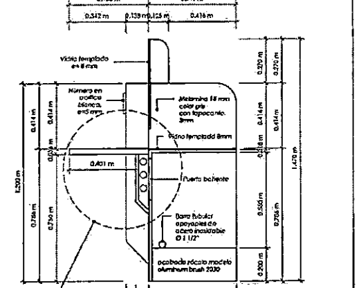
CORTE B-B ESC: 1/15
