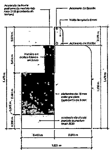
ELEVACION LATERAL 01 ESC: 1/15
