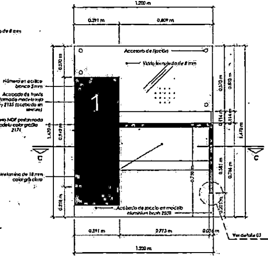
ELEVACION FRONTAL ESC: 1/15
