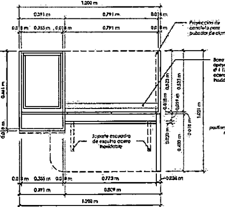
CORTE C-C ESC: 1/15
