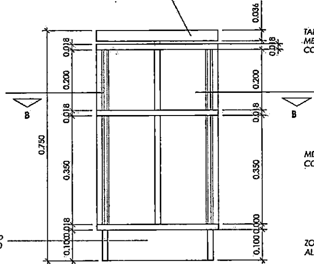
CORTE A-A
