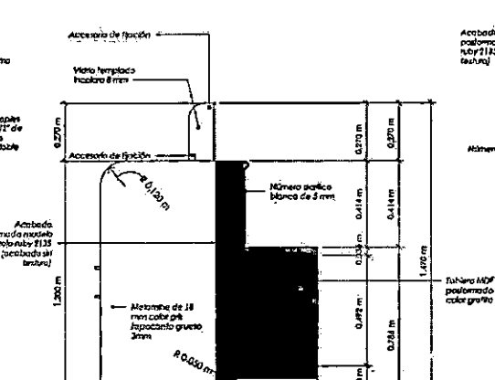
ELEVACION LATERAL 02 ESC: 1/15
