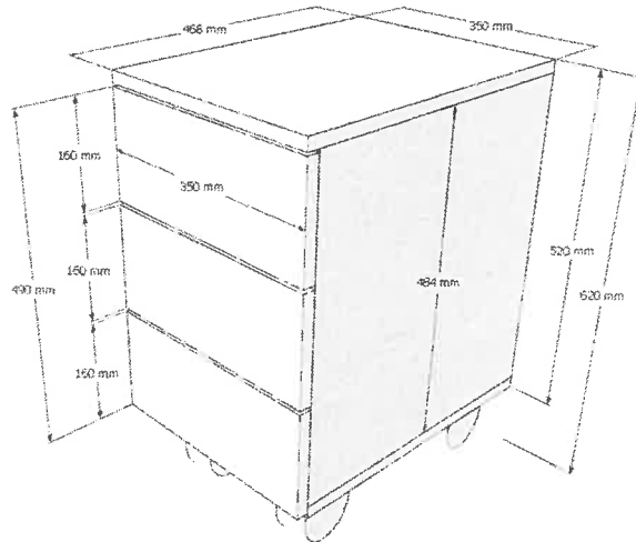
Cajonera móvil
