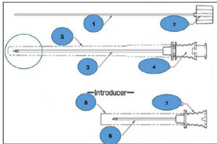
Fig. 1: Aguja espinal con introductor (no incluye diseño)
