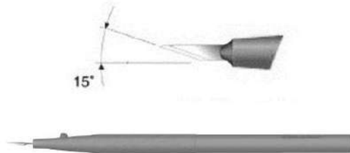
Fig.1: Cuchillete de 15° para cirugía oftalmológica (no incluye diseño)
