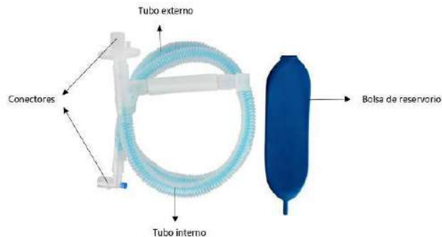
Fig.1: Circuito de anestesia coaxial (no incluye diseño)
