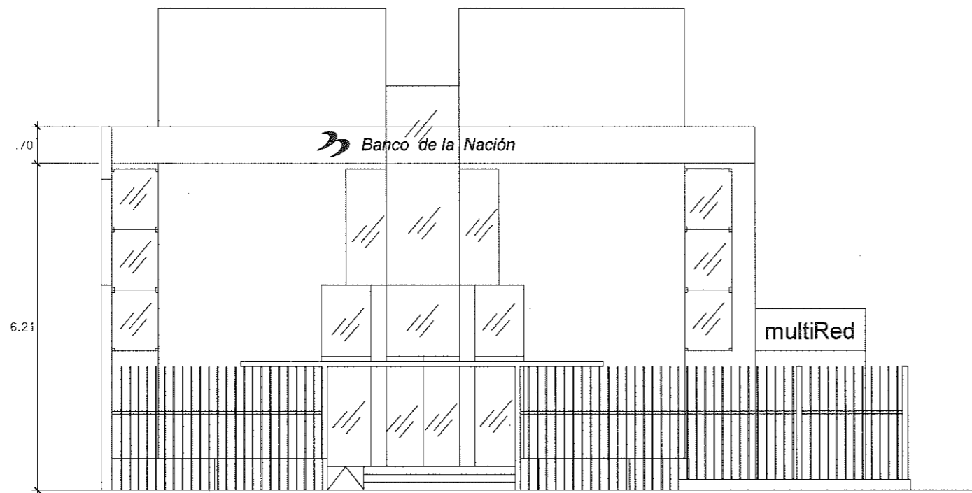
ELEVACION PRINCIPAL
