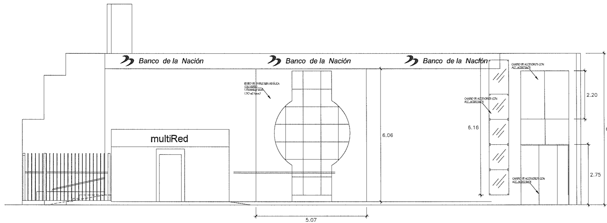
ELEVACION LATERAL
