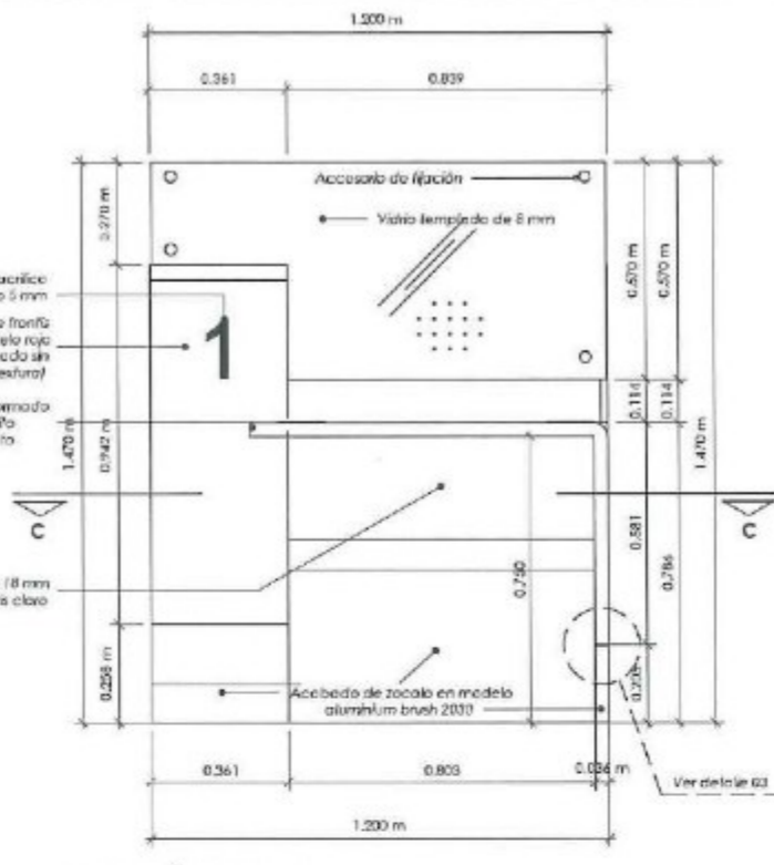
ELEVACIÓN FRONTAL ESC: 1/15
