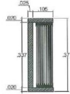
ELEVACIÓN LATERAL
