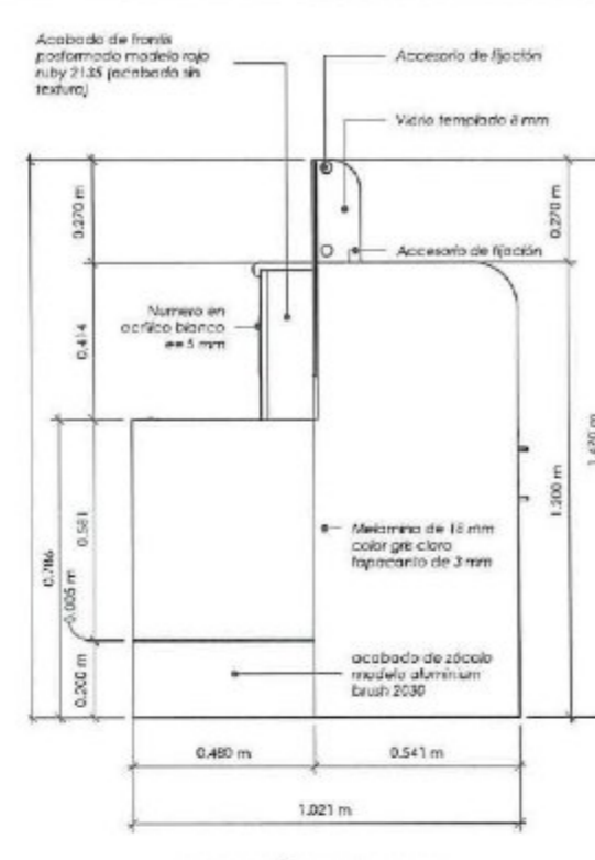
ELEVACIÓN LATERAL 01 ESC: 1/15
