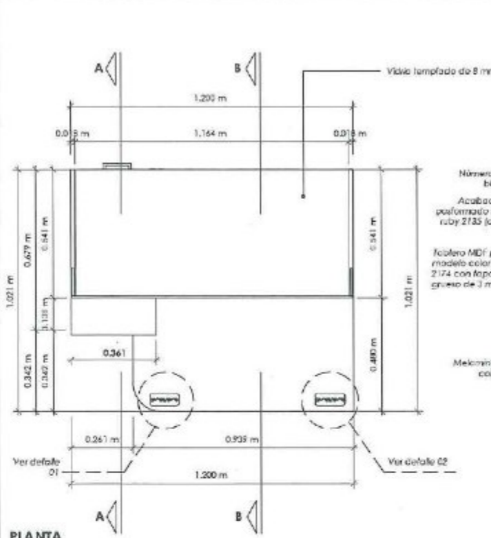
PLANTA ESC: 1/15
