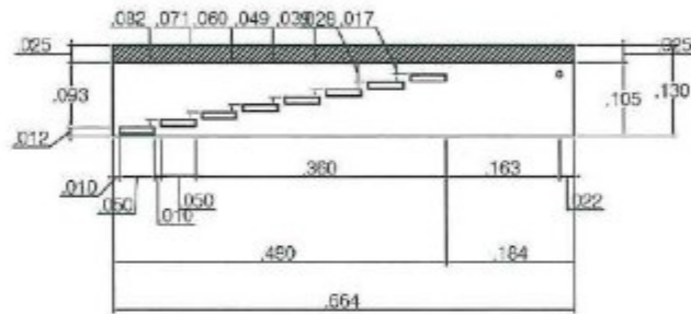
SECCIÓN 1-1
