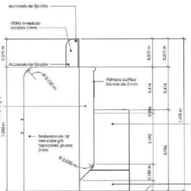
ELEVACIÓN LATERAL 02 ESC: 1/15
