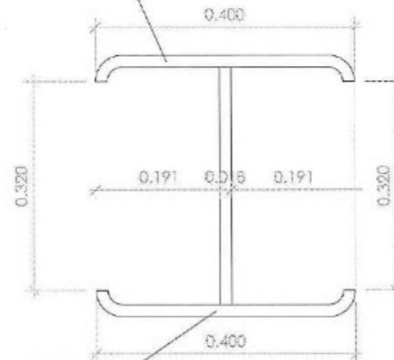
CORTE B-B
