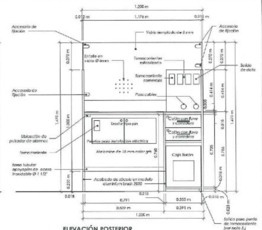
ELEVACIÓN POSTERIOR ESC: 1/15
