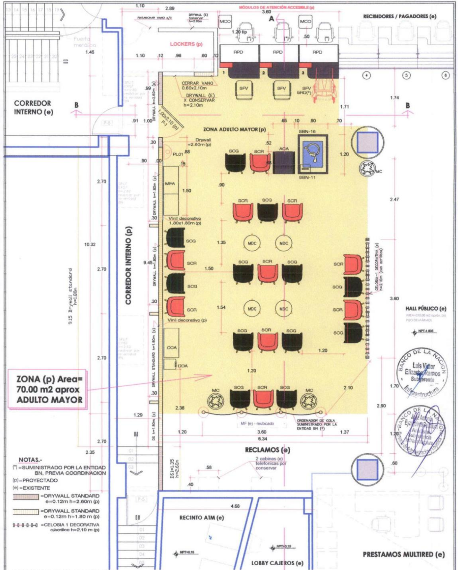
PLANTA PROPUESTA ADULTO MAYOR - AG1 TRUJILLO
