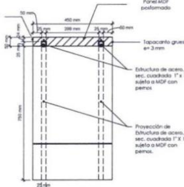
CORTE C-C ESC: 1/10
