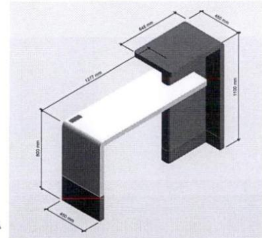
DETALLE 04
