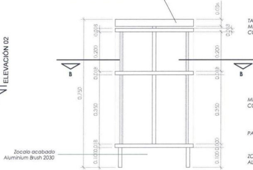
CORTE A-A
