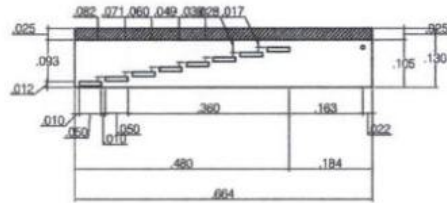
SECCIÓN 1-1
