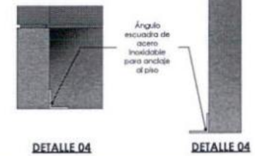
DETALLE 04
