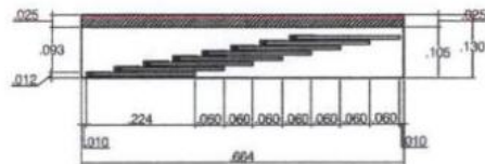
SECCIÓN 2-2
