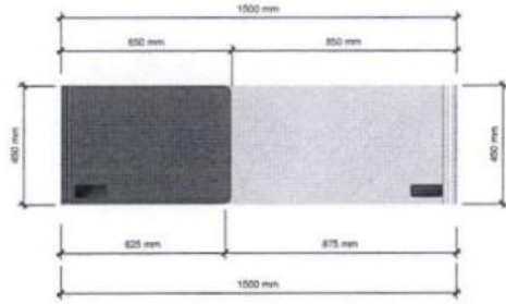
PLANTA ESC: 1/15
