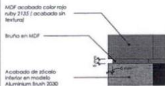
DETALLE 02 ESC: 1/2
