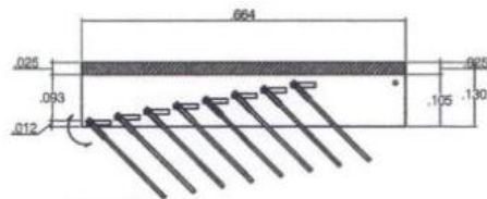
SECCIÓN 2-2
