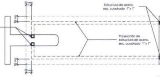
CORTE B-B ESC: 1/10
