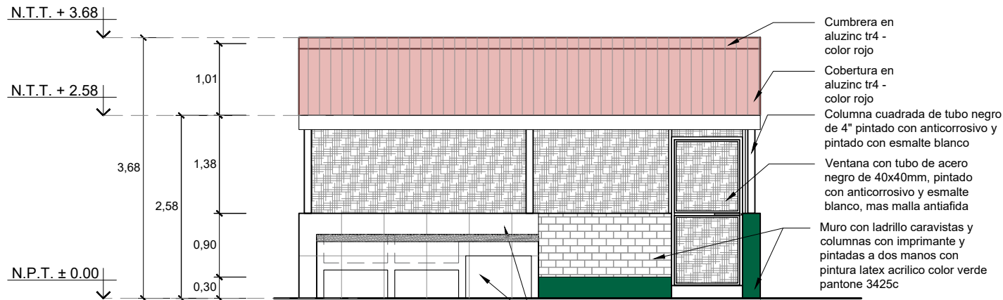
ELEVACION FRONTAL ESC. 1/75
