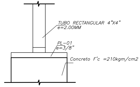
DETALLE DE APOYO DE COLUMNA ESC. 1/10
