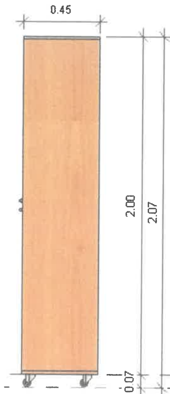
VISTA LATERAL
