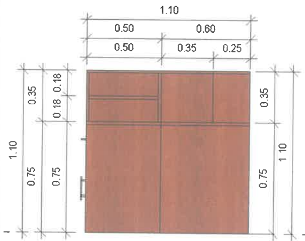
VISTA LATERAL
