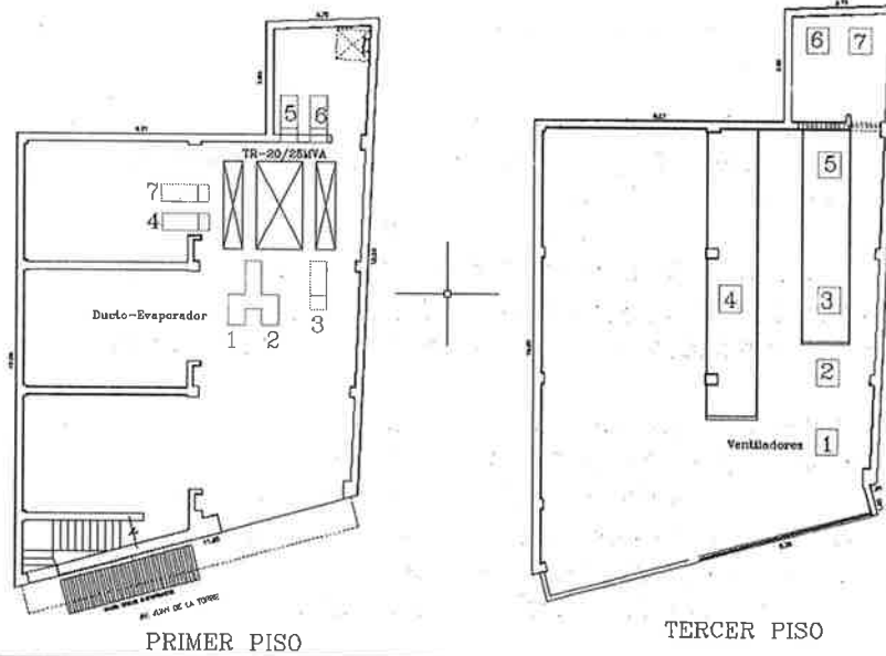
Plano 1: ubicación de los equipos
