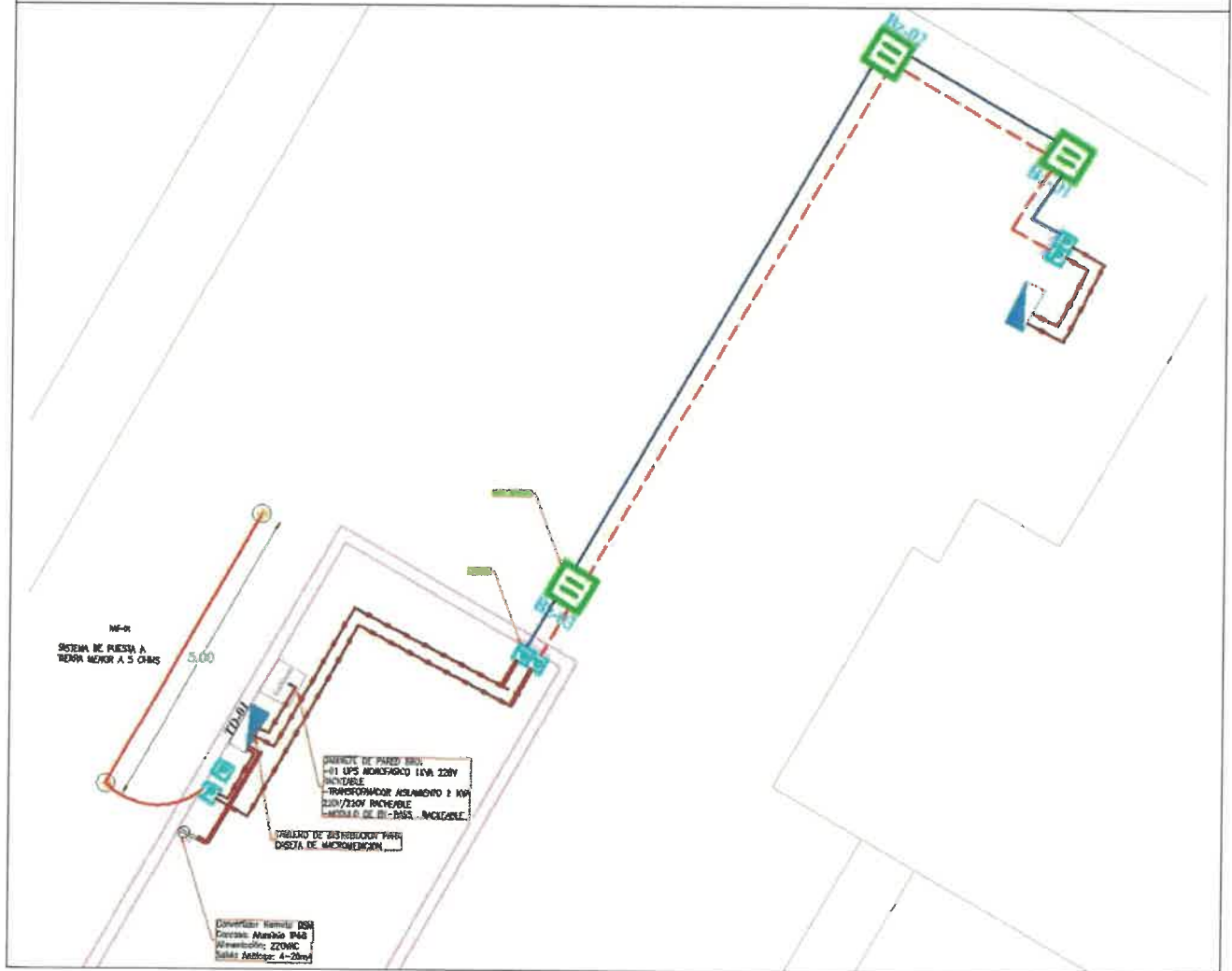
Ubicación propuesta de medidores de caudal al interior de la cámara
