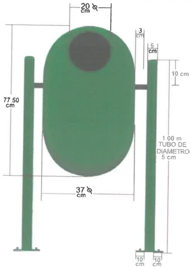
Imagen 1. Medidas del tacho unitario
