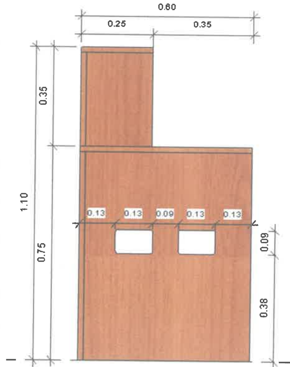
CORTE 1-1
