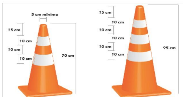
Figura 5.3 Ejemplo de conos con dimensiones
