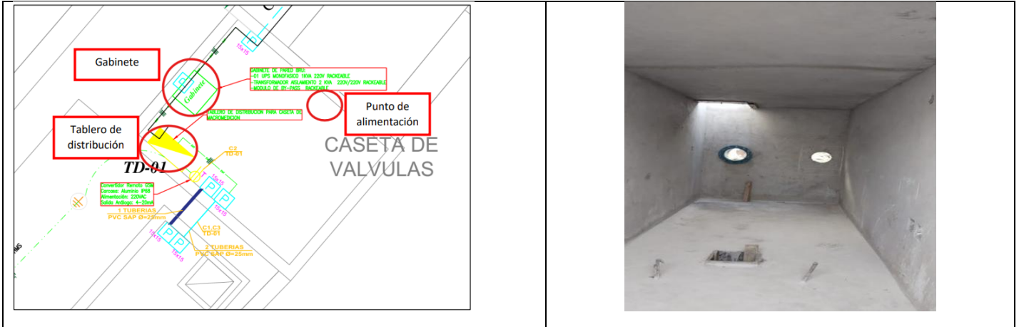
Ubicación propuesta de medidores de caudal al interior de la cámara
