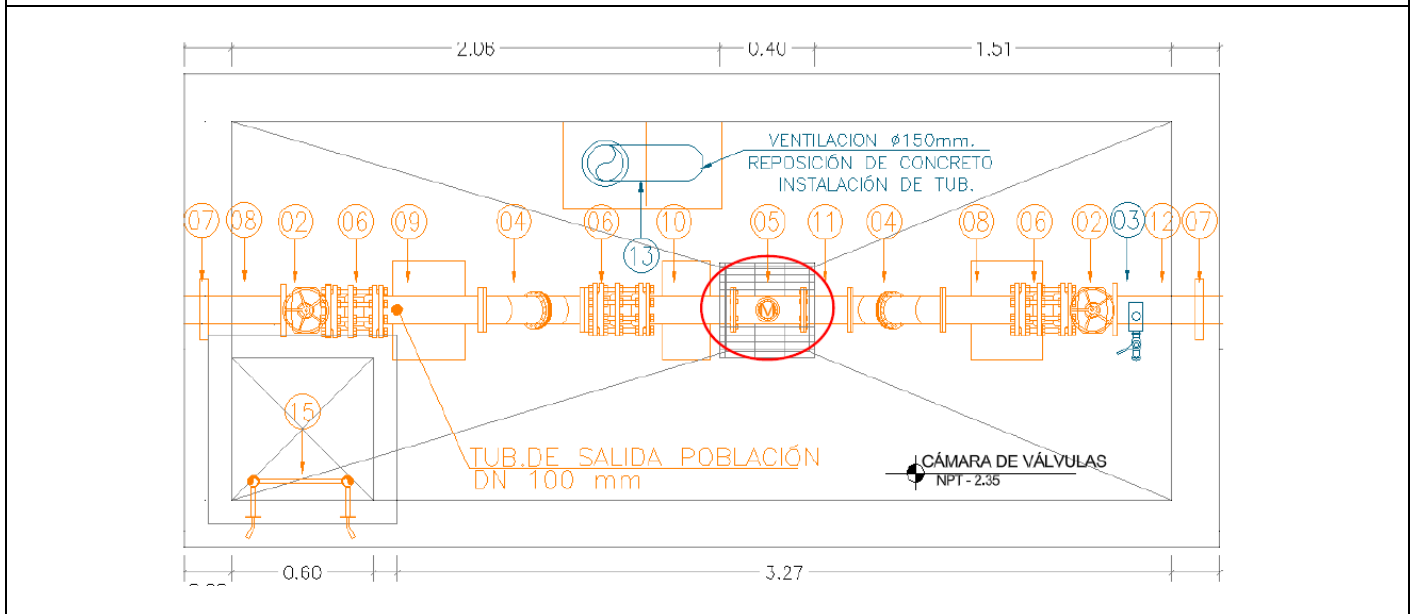
Ubicación propuesta de medidores de caudal al interior de la cámara
