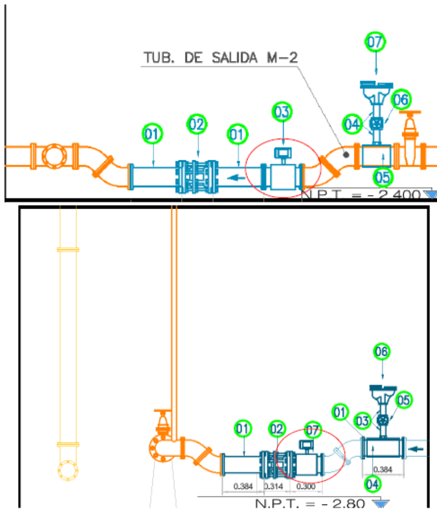
Ubicación propuesta de medidores de caudal al interior de la cámara
