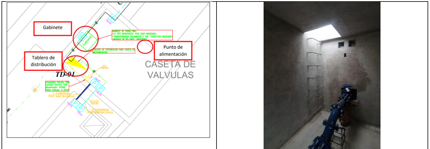
Ubicación propuesta de medidores de caudal al interior de la cámara
