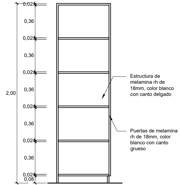
CORTE 01 ESC. 1/25
