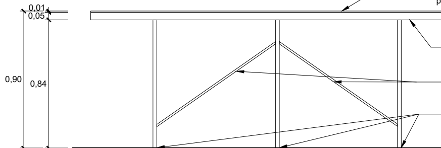
ELEVACION FRONTAL
