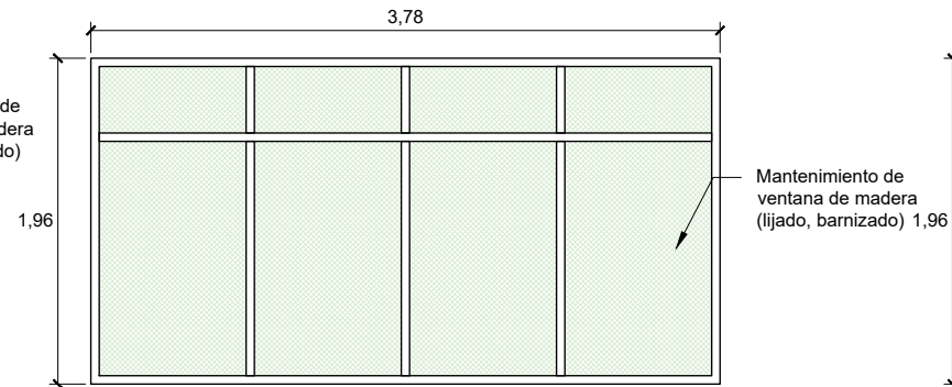
V-07 (Pabellon A) ESC. 1/50
