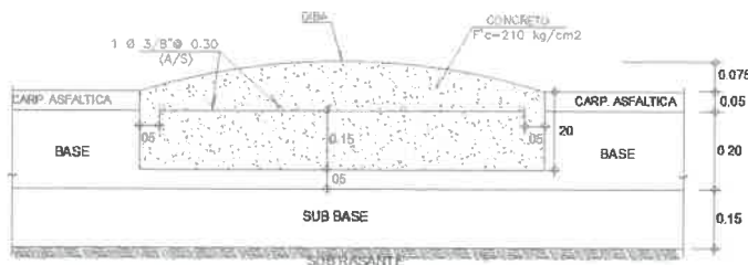
DETALLE ESTRUCTURAL ESC. 1/10
