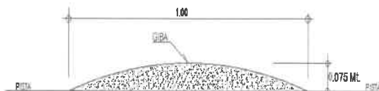
CORTE B-B ESC. 1/10
