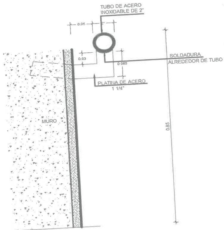
DETALLE - 2 ESC. 1/2
