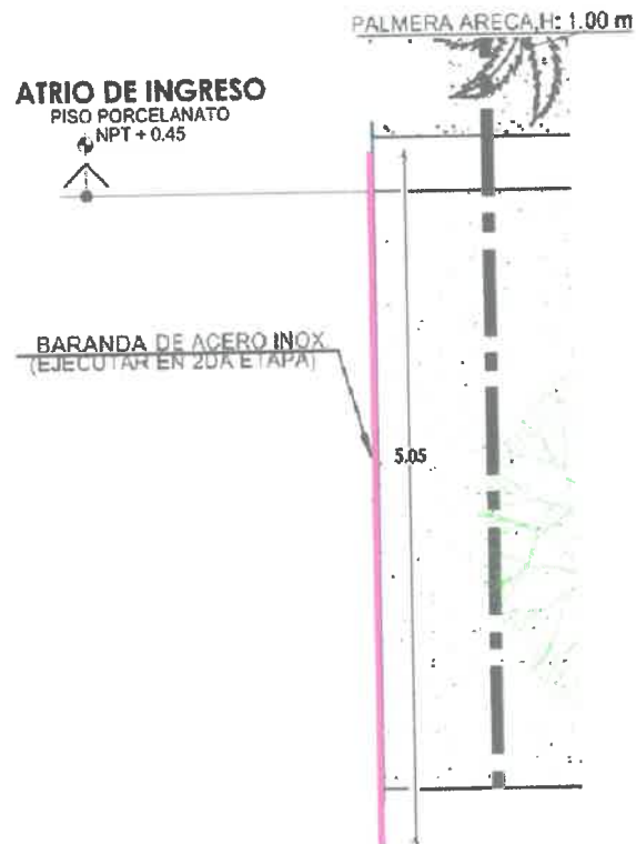
Fig.09. Vista de planta de baranda
