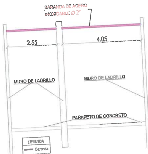
Fig.04. Vista de planta de modelo 2 y modelo 3 de baranda de acero inoxidable
