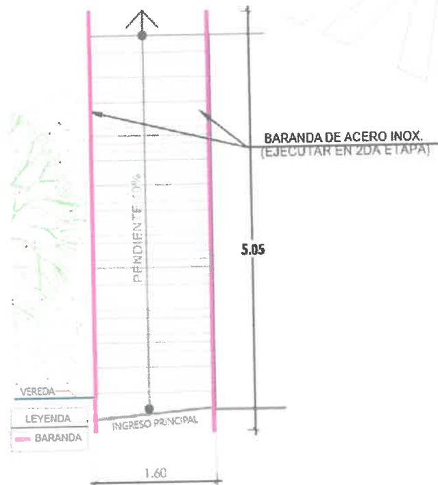
Fig.08. Vista de planta de baranda
