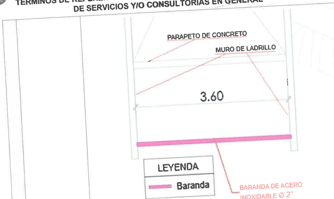
Fig.03. Vista de planta de modelo 1 de baranda de acero inoxidable
