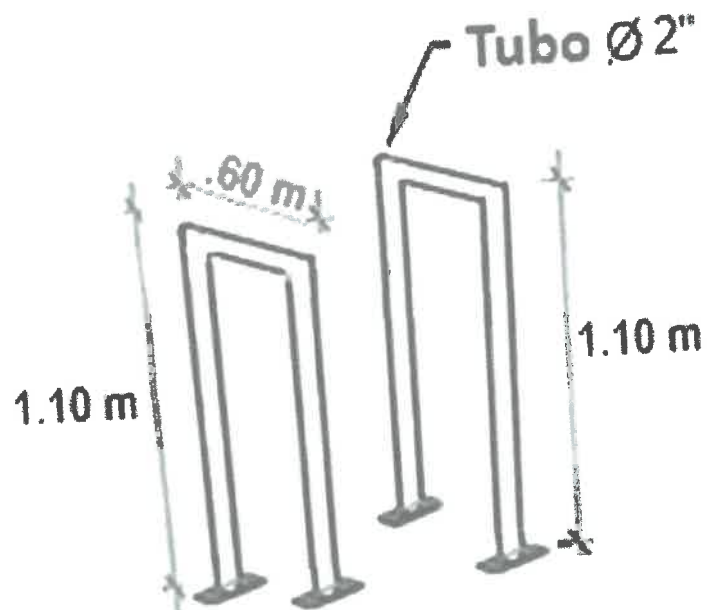
Fig.02. Vista Isométrica de pasamano de la escalera de gato
