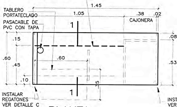
PLANTA ESC: 1/20
