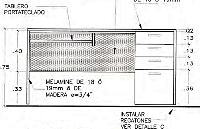
ELEVACION ESC: 1/20
