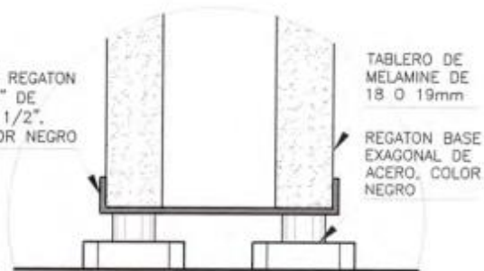
DETALLE C' ESC: 1/2
