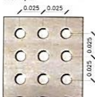
DETALLE E PLANCHA DE ACERO PERFORADA ESC: 1/2
