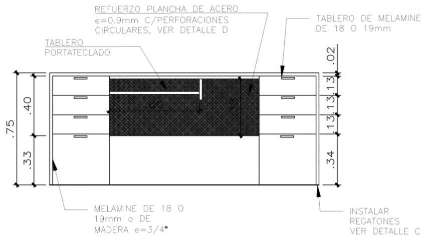
ELEVACIÓN ESC: 1/20
