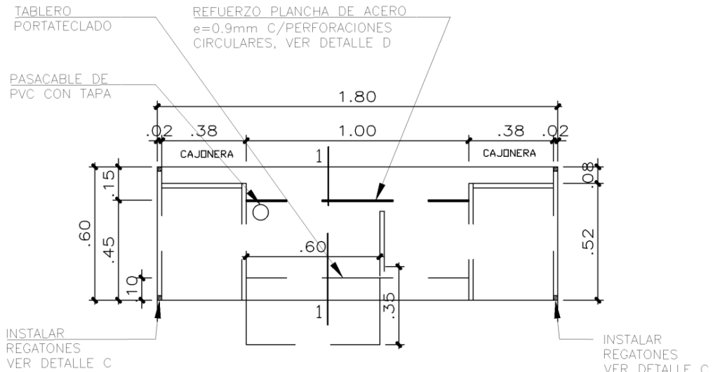
PLANTA ESC: 1/20
