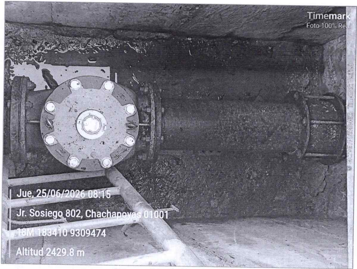
Macromedidor de 200 mm (8")
