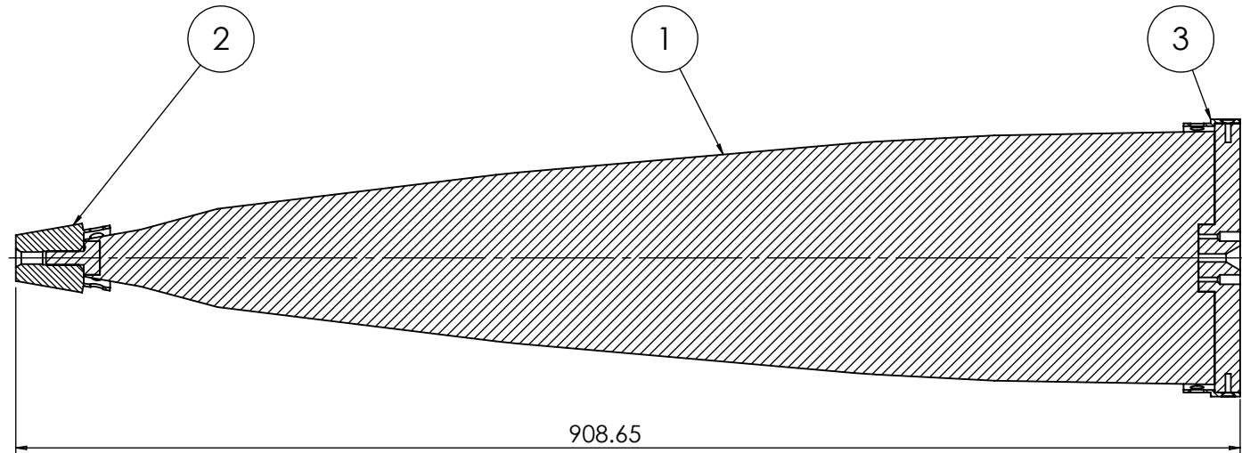
SECCIÓN A-A ESCALA 1 : 5
