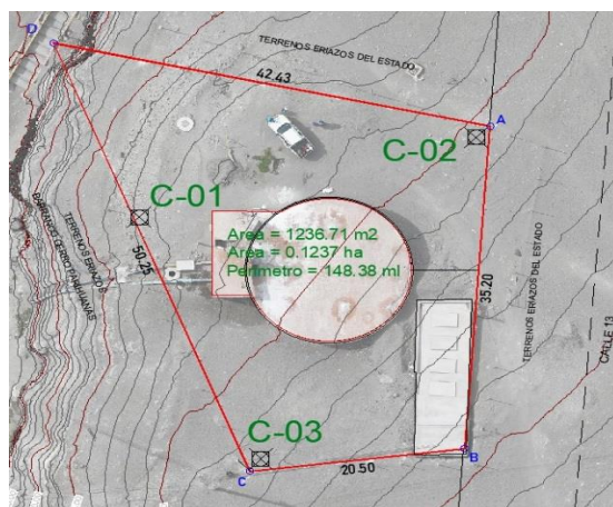
Ilustración 2 Reservoir R-02
