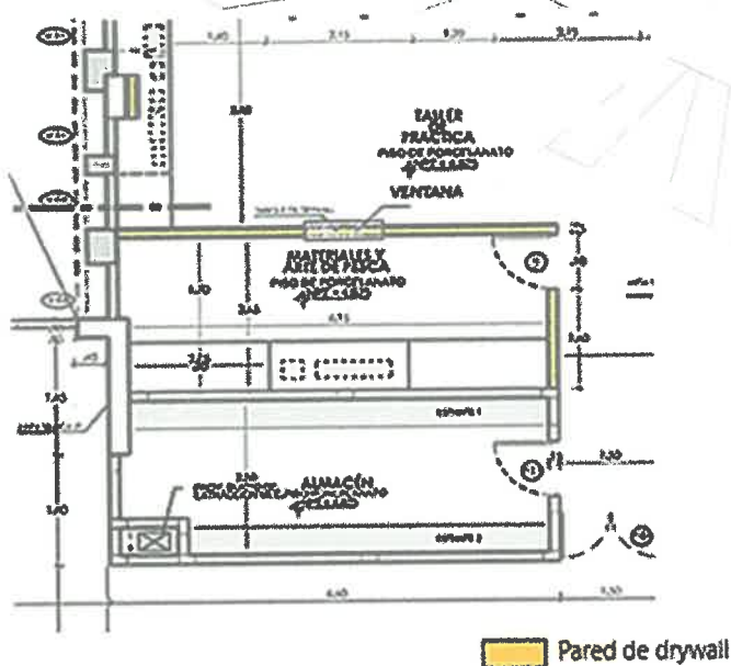
Fig.3. Plano de ubicación de la ventana fija
