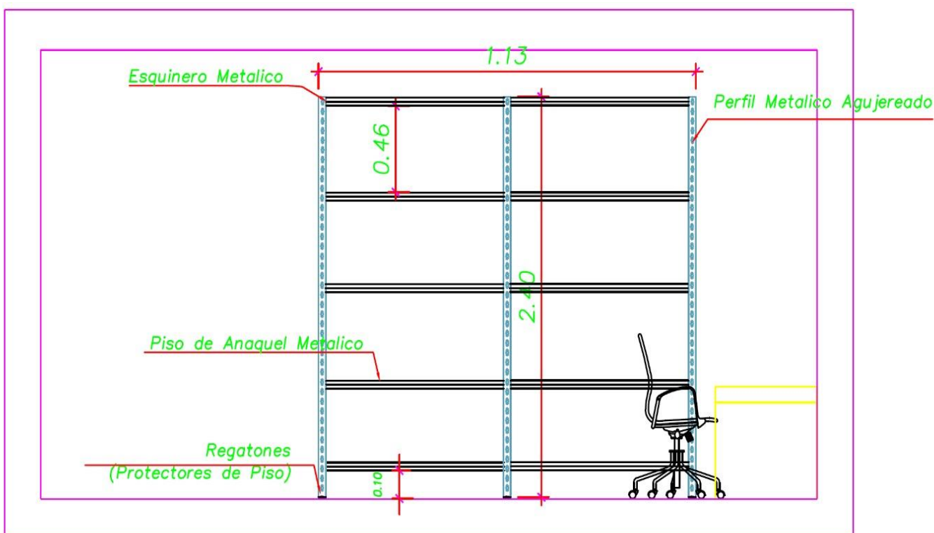
CORTE A-A
