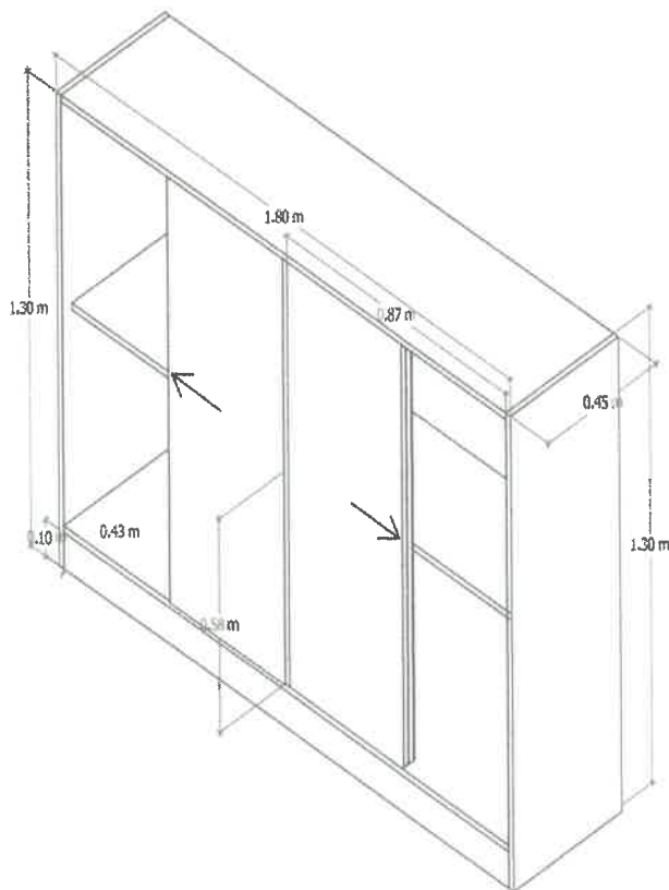
VISTA ISOMETRICA
