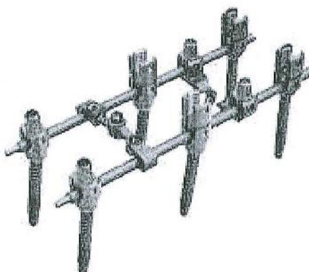
Fig.1: Set de fijación transpedicular para columna vertebral (No incluye diseño)
