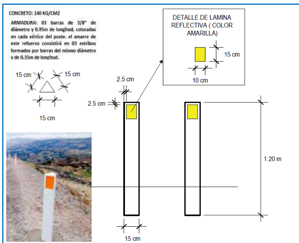
Imagen 01: Dimensiones e imagen referencial del Poste Delineador
