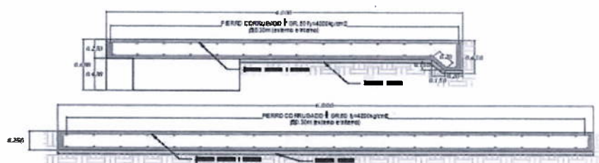
DETALLE LOSA DE APROXIMACION
