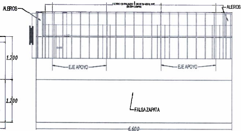
DETALLE PARAPETO
