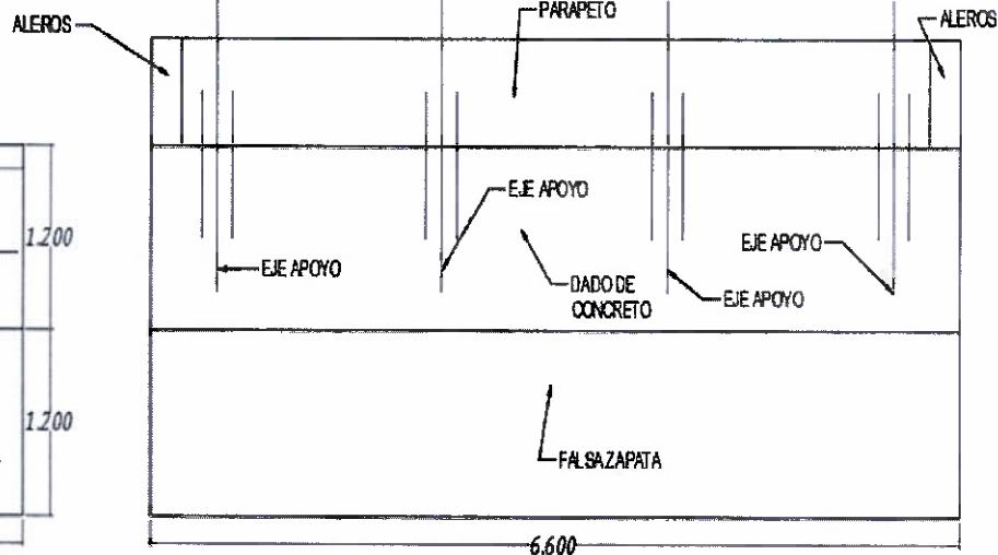
DETALLE APOYOS
