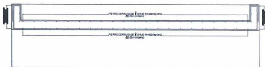
DETALLE LOSA DE PARAPETO
