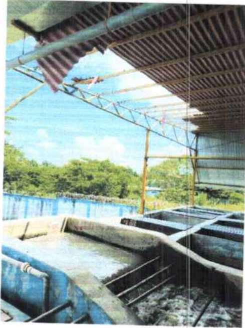
Imagen 1. Imagen lado izquierdo. Zona de Mezcla Rápida y Floculador
