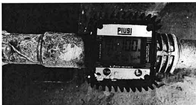
Medidor N° 5: Atico - Medidor entrada grupo electrógeno, para Perkins 3 (de 1")
