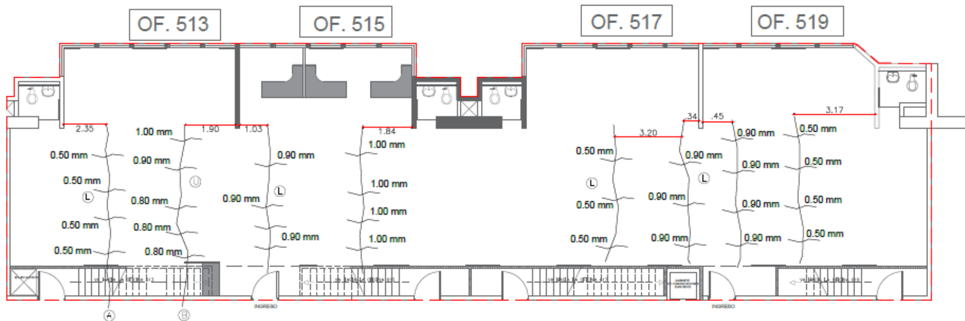
PLANO DE FISURAS EN TECHOS
