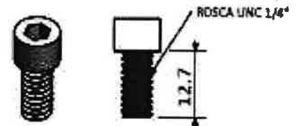
DETALLE "F" PERNO SOCKET UNC 1/4" X 1/2" 3 UND
