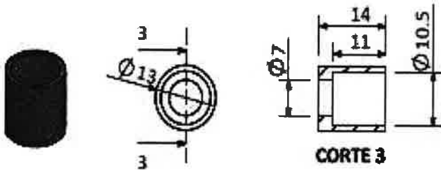
DETALLE "E" BOCINA 2 UND
