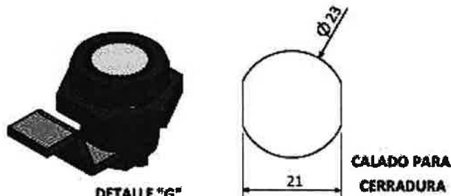
DETALLE "G" CERRADURA DE BÓNC RANURADA 36 DIENTES 1 UND
